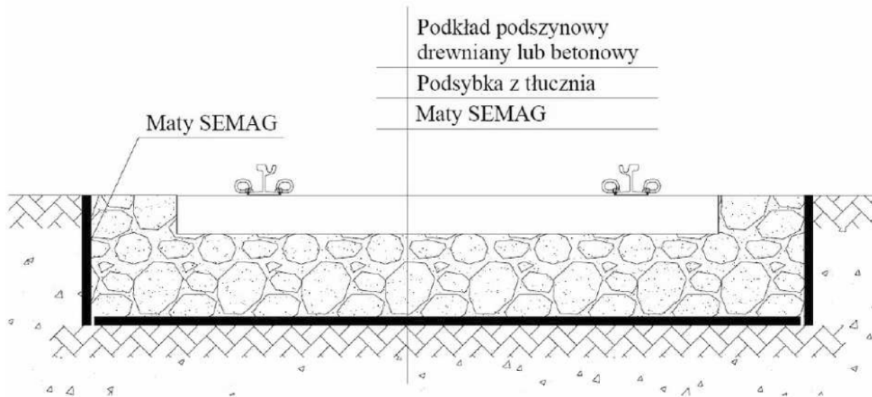
Rysunek Z-1- Przekrój poprzeczny stosowania maty MW SEMAG
